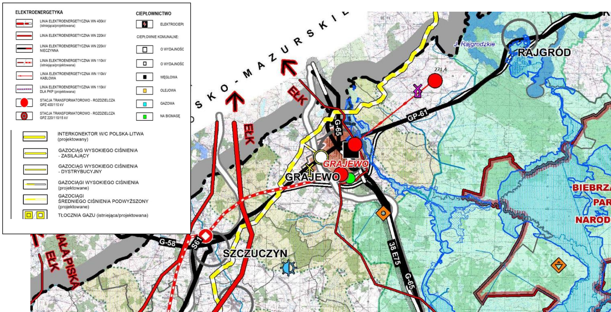
Rys. nr 17.3 Alokacja planowanych linii energetycznych i gazowych między miastem Grajewo, a gminami ościennymi. Źródło: Plan Zagospodarowania Przestrzennego Województwa Podlaskiego.
