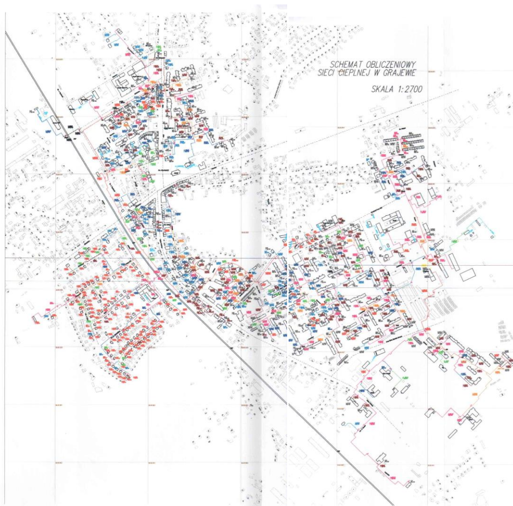
Rysunek nr 7.2 schemat sieci ciepłowniczej na terenie Grajewa
