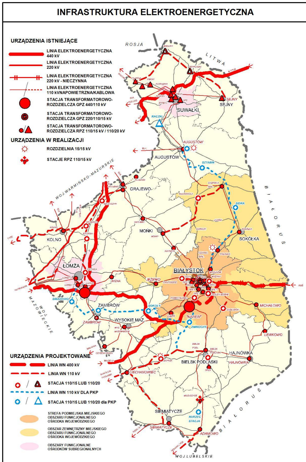
Rys. nr 9.2 infrastruktura elektroenergetyczną na terenie województwa podlaskiego Źródło: PLAN ZAGOSPODAROWANIA PRZESTRZENNEGO WOJEWÓDZTWA PODLASKIEGO
