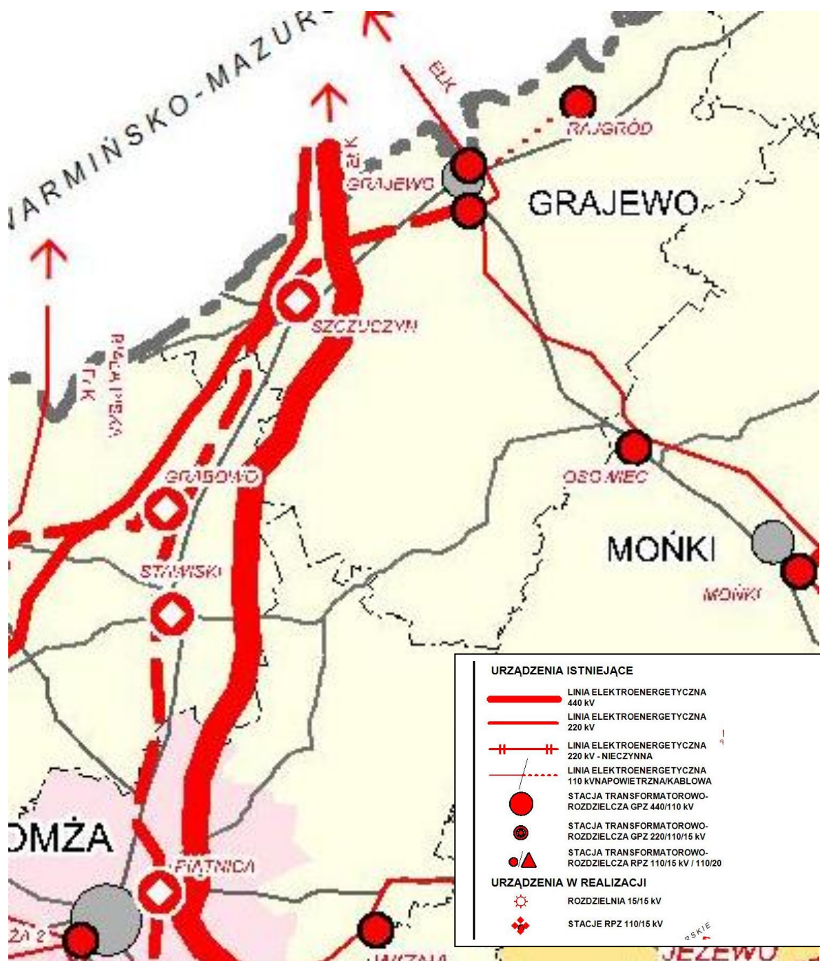
Rys. nr 17.2 Alokacja planowanych linii energetycznych w obszarze miasta Grajewo. Źródło: Plan Zagospodarowania Przestrzennego Województwa Podlaskiego.
