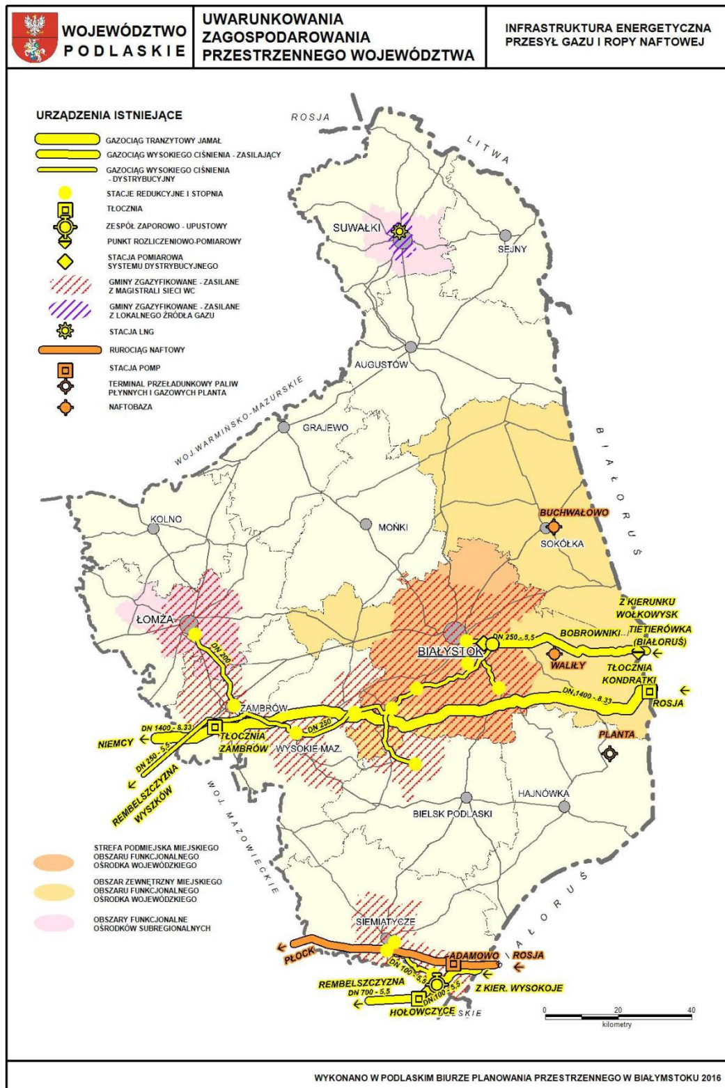
Rys. nr 8.1 infrastruktura energetyczna przesyłu gazu na terenie województwa podlaskiego. Źródło: PLAN ZAGOSPODAROWANIA PRZESTRZENNEGO WOJEWÓDZTWA PODLASKIEGO.
