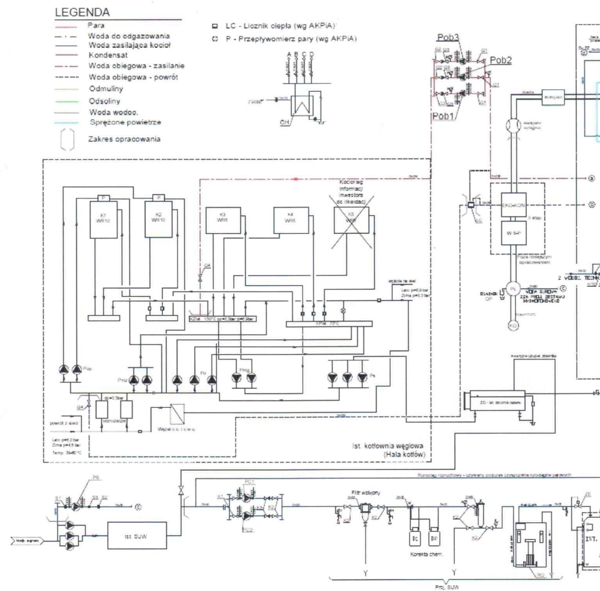
Schemat jednostki kogeneracyjnej zainstalowanej w PEC w Grajewie
